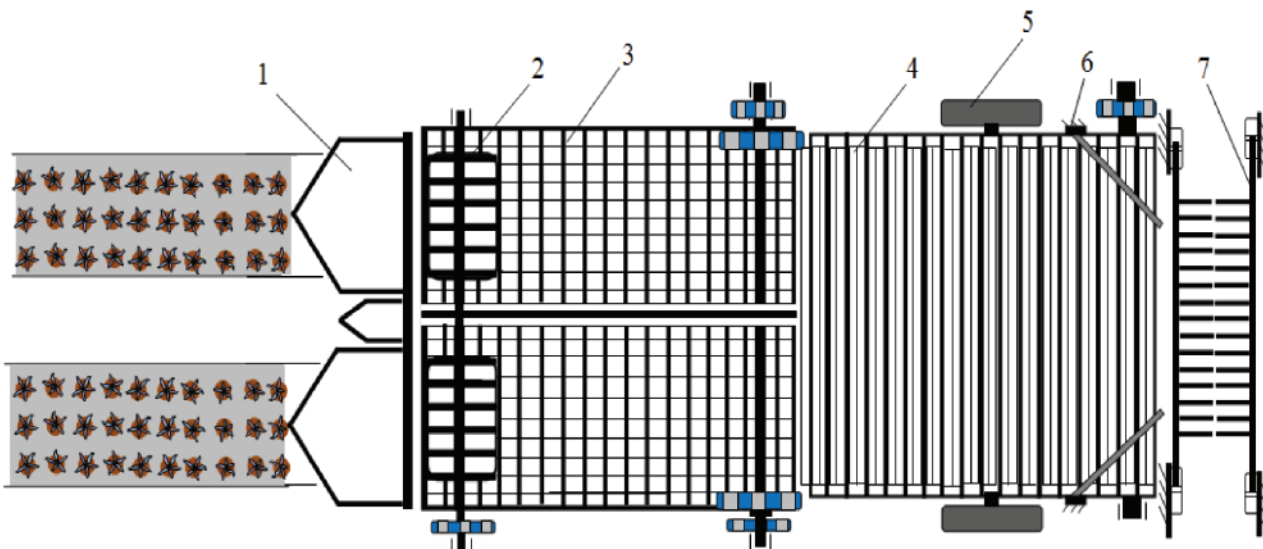
1-рasm. Сабзи ковлагич конструктив схемаси:
