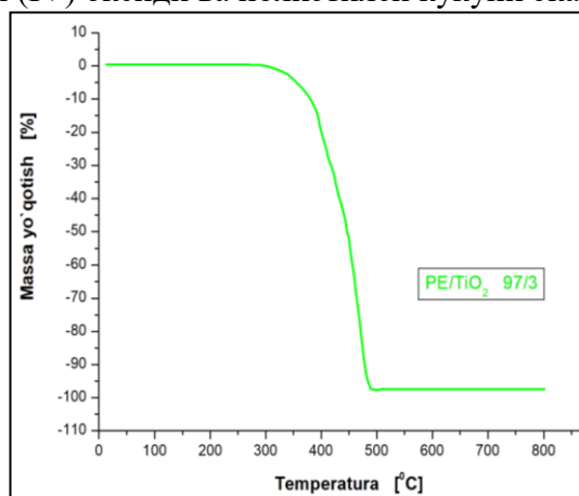
15-расм. PE:TiO_2=97/3 нисбатда олинган намуналарнинг ТГ эгри чизиги (температура ортиши билан масса йўқолиб бориш графиги)
