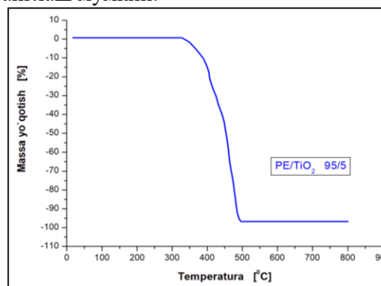
16-расм. PE:TiO_2=95/5 нисбатда олинган намуналарнинг ТГ эгри чизиги (температура ортиши билан масса йўқолиб бориш графиги)
