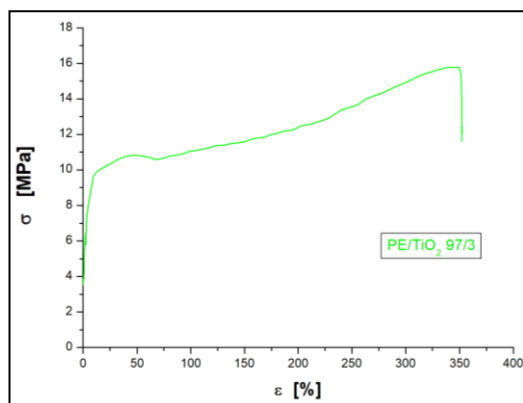
3-расм. Таркибида 97% F-0320 маркали қуйи зичликли чизиқли полиэтилен ва 3% титан (IV) оксиди бўлган композицион материални чўзишда кучланиш ( \sigma ) нинг нисбий деформация ( \epsilon ) га боғлиқлиги
