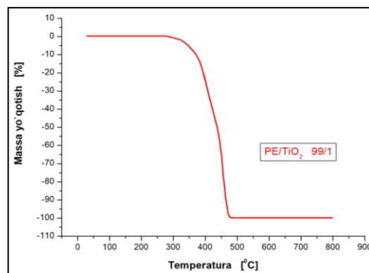
14-расм. PE:TiO_2=99/1 нисбатда олинган намуналарнинг ТГ эгри чизиги (температура ортиши билан масса йўқолиб бориш графиги)
