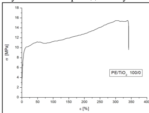
1-расм. F-0320 маркали қўйи зичликли чизикли полиэтиленни чўзишда кучланиш ( \sigma ) нинг нисбий деформация ( \epsilon ) га боғлиқлиги
