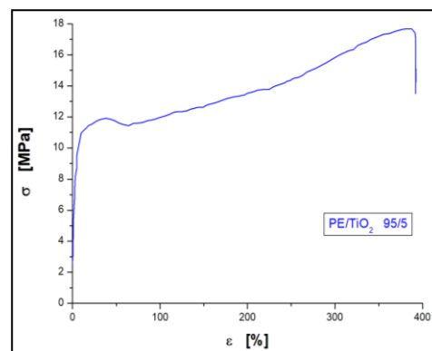
4-расм. Таркибида 95% F-0320 маркали қуйи зичликли чизиқли полиэтилен ва 5% титан (IV) оксиди бўлган композицион материални чўзишда кучланиш ( \sigma ) нинг нисбий деформация ( \epsilon ) га боғлиқлиги
