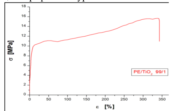
2-расм. Таркибида 99 % F-0320 маркали қўйи зичликли чизикли полиэтилен ва 1 % титан (IV) оксиди бўлган композицион материални чўзишда кучланиш ( \sigma ) нинг нисбий деформация ( \epsilon ) га боғлиқлиги
