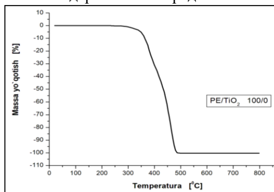
13-расм. PE:TiO_2=100/0 нисбатда олинган намуналарнинг ТГ эгри чизиги (температура ортиши билан масса йўқолиб бориш графиги)
