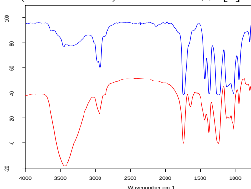
6-расм. F-0320 маркали қуйи зичликли чизиқли полиэтилен ва титан (IV) оксиди таркибли композицион плёнкасининг ИҚ-спектрлари 7-расм. F-0320 маркали қуйи зичликли чизиқли полиэтилен ва титан (IV) оксиди таркибли композицион материаллар плёнкасининг ИҚ-спектрлари
