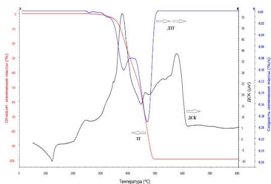
8-расм. F-0320 маркали қуйи зичликли чизиқли полиэтиленнинг TG, DTG, DSC эгри чизиқлари
