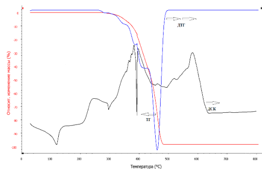
9-расм. Таркибида 99% F-0320 маркали қуйи зичликли чизиқли полиэтилен ва 1% титан (IV) оксиди бўлган композицион материалнинг TG, DTG, DSC эгри чизиқлари
