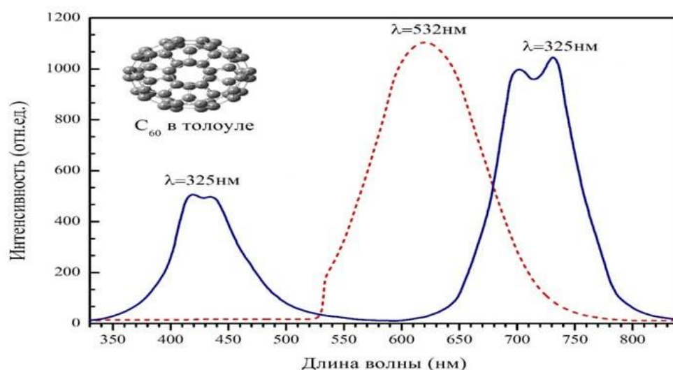
Рис. 1. Спектры флуоресценции раствора C 60 в толуоле с концентрацией 0,1 г/л: сплошная линия — возбуждение УФ-излучением ( \lambda = 325 нм), штриховая линия — возбуждение видимым излучением ( \lambda = 532 нм)
