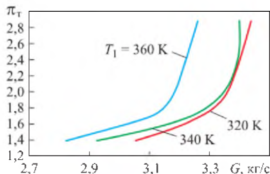
2-rasm. Gazning oʻzgaruvchan boshlangʻich harorati sharoiti uchun turbodetander tavsifnomalari.
