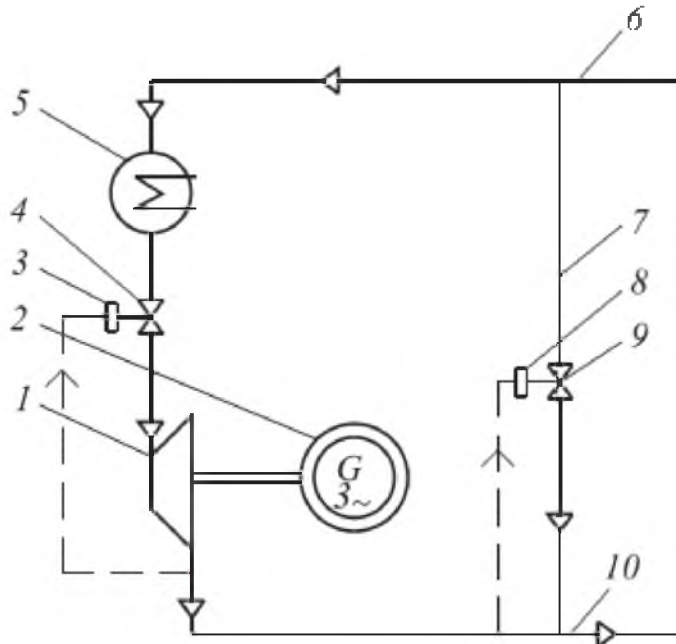
1-rasm. Detander-generator qurilmasining prinsipial sxemasi.
