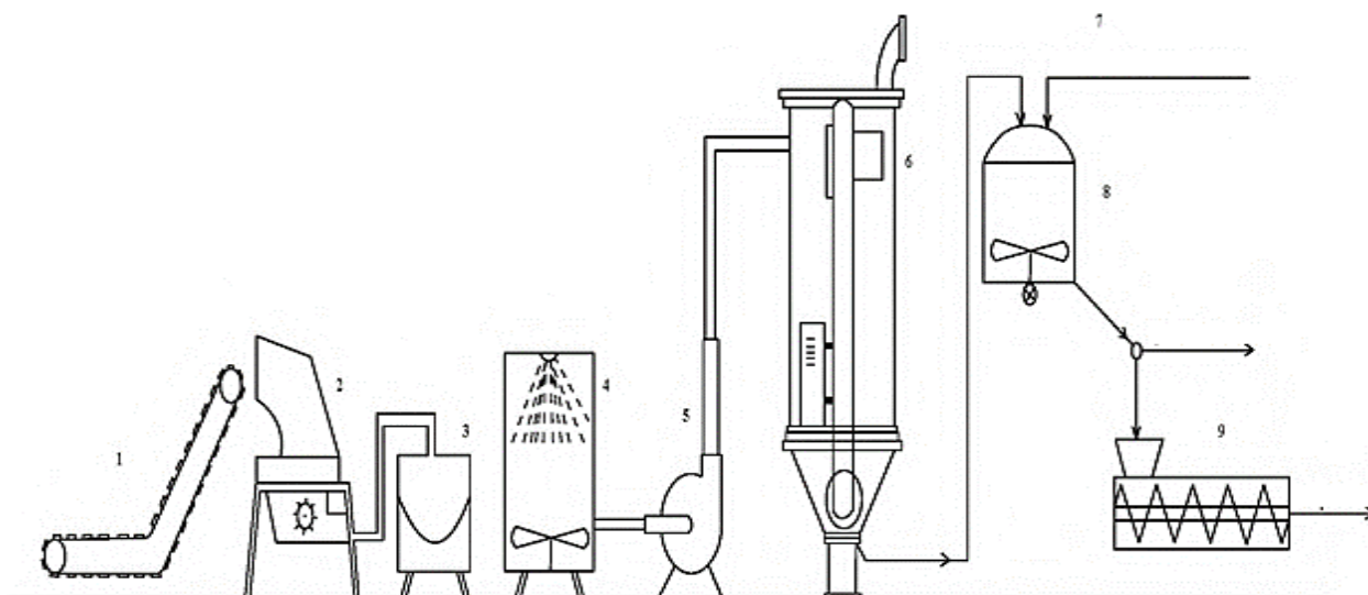
1 – сортировочный участок; 2 – дробилка; 3 – магнитный уловитель; 4 – мойка; 5 – центрифуга; 6 – сушильное устройство; 7 – участок добавления пластификатора; 8 – смеситель; 9 – гранулятор
