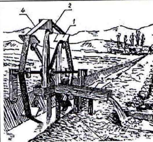
5-расм. Чархпалак.
